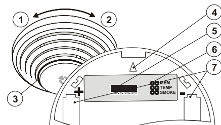
Fig 6: 1– apertura de la tapa del detector; 2 – cierre de la tapa del detector; 3 – señal óptica de estado; 4 – flecha que muestra dónde insertar el detector; 5 – código de producción; 6 – terminales de configuración; 7 – soporte para pilas;
